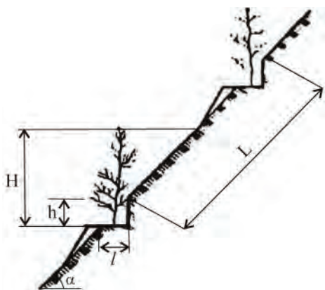
Профиль ступенчатых площадок на горном склоне: H – высота деревьев, м; h – глубина вертикального вреза площадки, м; l – ширина горизонтального вреза полотна площадки; \alpha – крутизна склона; L – расстояние между площадками.
