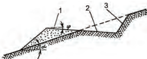
Схема выемочно-насыпной террасы:
